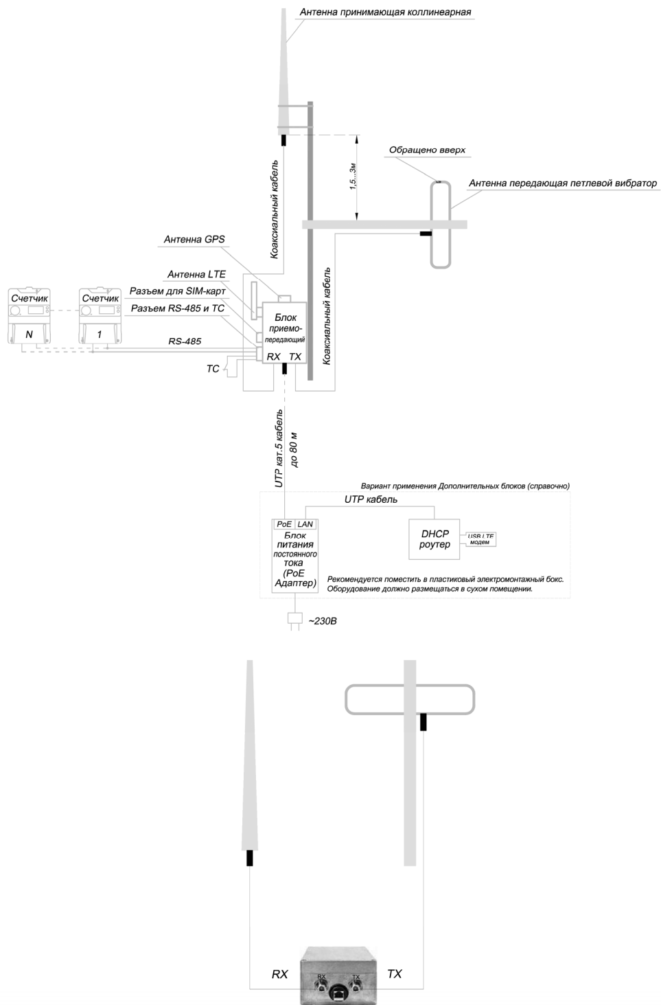
Рисунок А3 – Способ подключения Базовой станции
